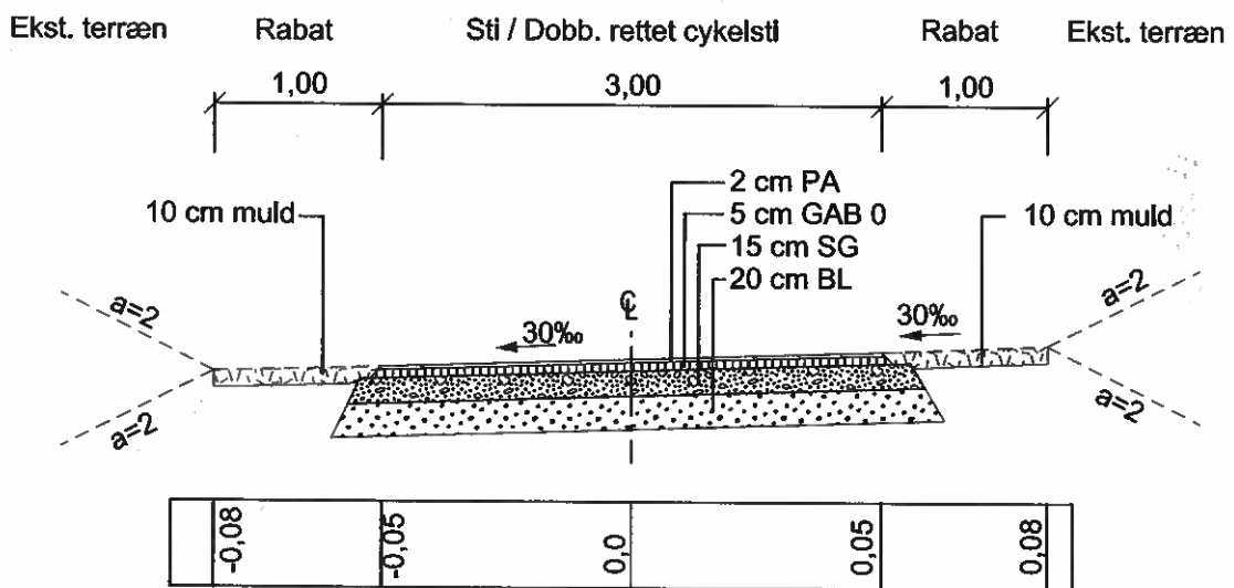
Normaltværprofil, 1:50
