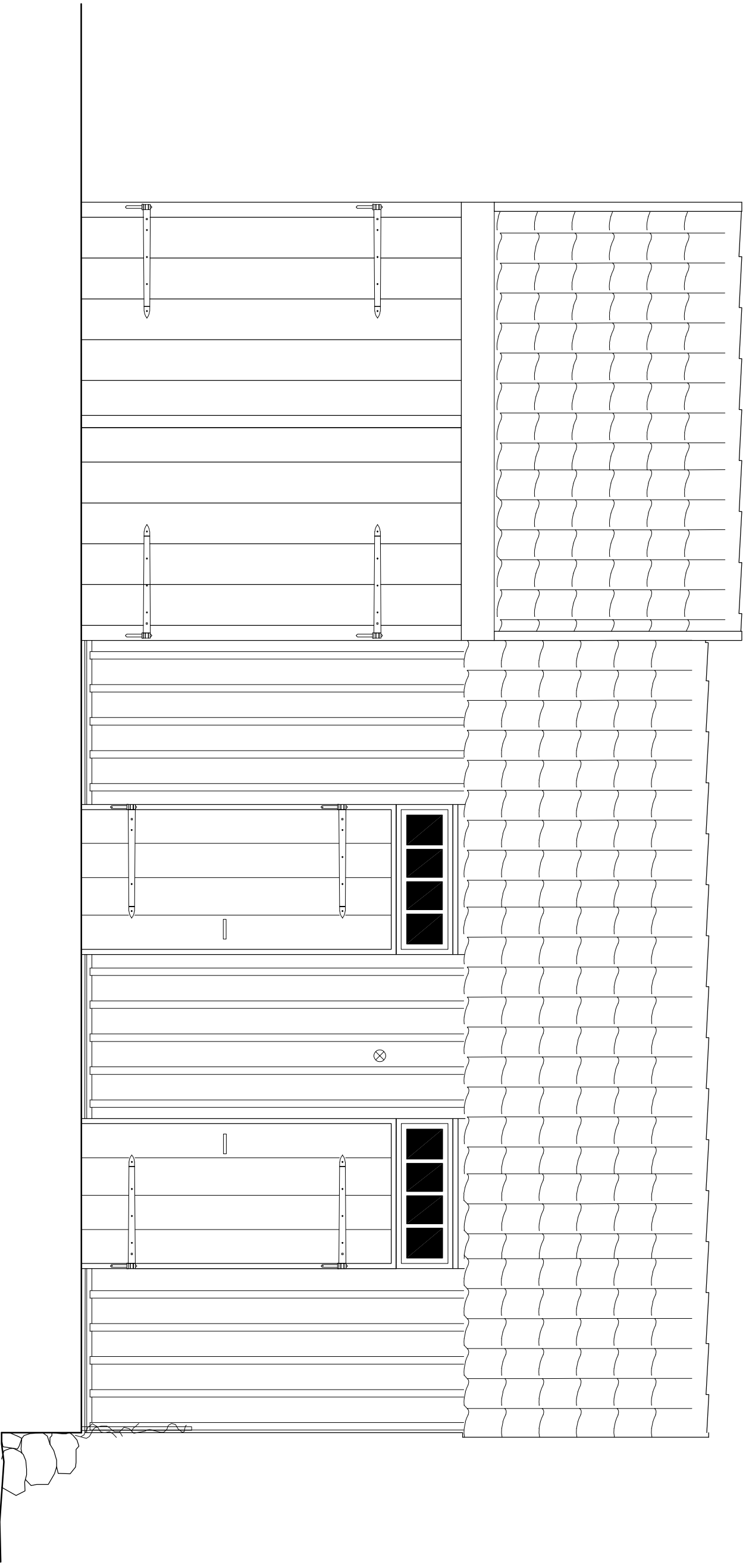
Nordfacade 1:50 Ny toilet bygning
