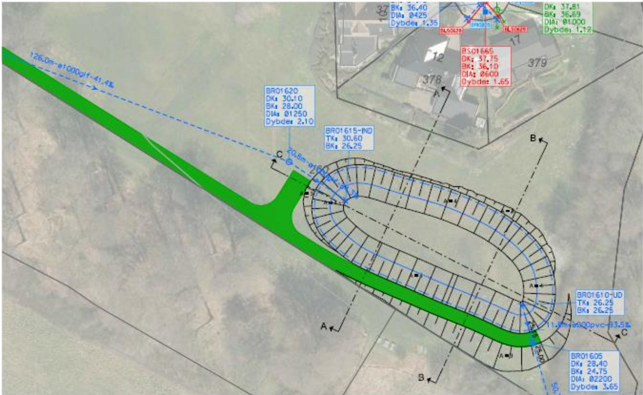
Skitse 1. Regnvandsbassin med en arealmæssig udbredelse ved permanent vandspejl på 1277m 2 og ved maksimalt vandspejl på 2109 m 2 . Det har et udløb til vandløbet på 24 l/s og terrænet etableres med anlæg på 1:3 og 1:4.
